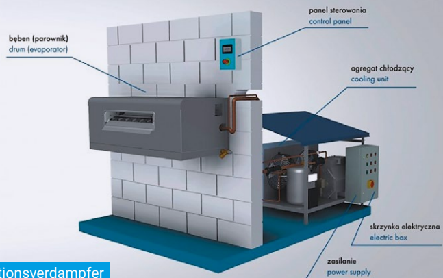
► Nowicki · Rotationsverdampfer
