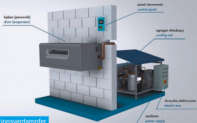
▶ Nowicki · Rotationsverdampfer
